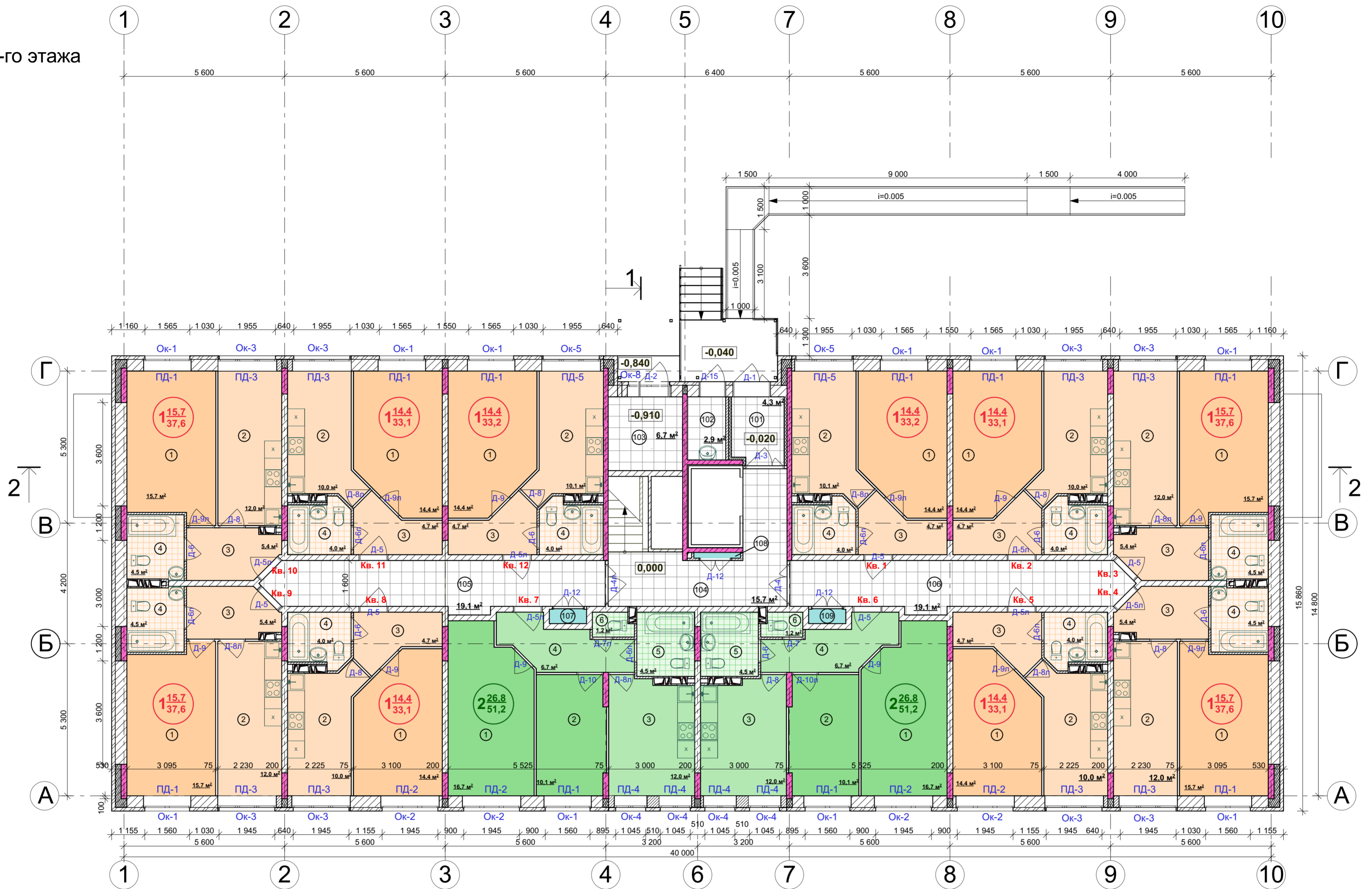
Экспликация помещений 1 этажа (начало)
