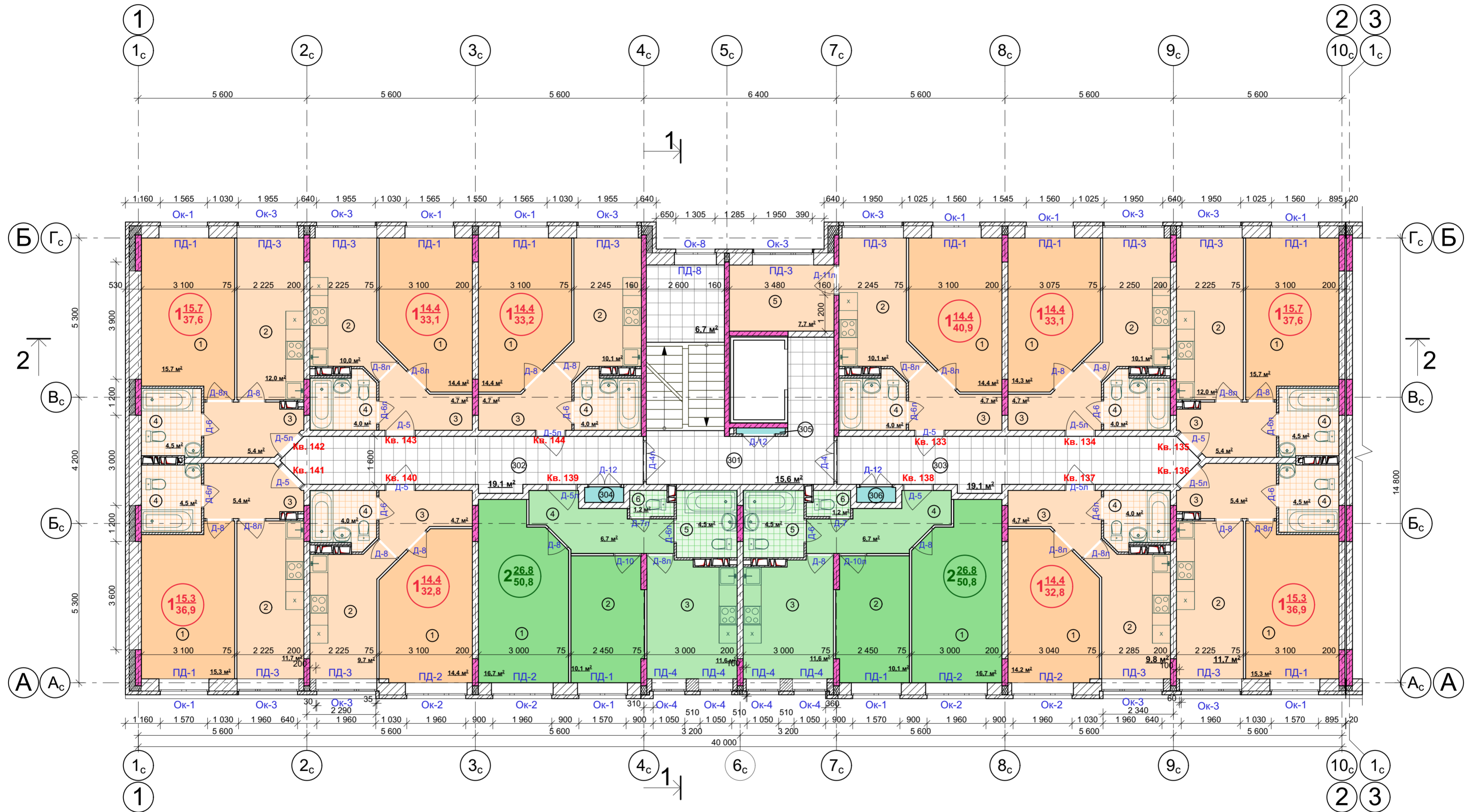
Экспликация помещений 3 этажа (начало)
