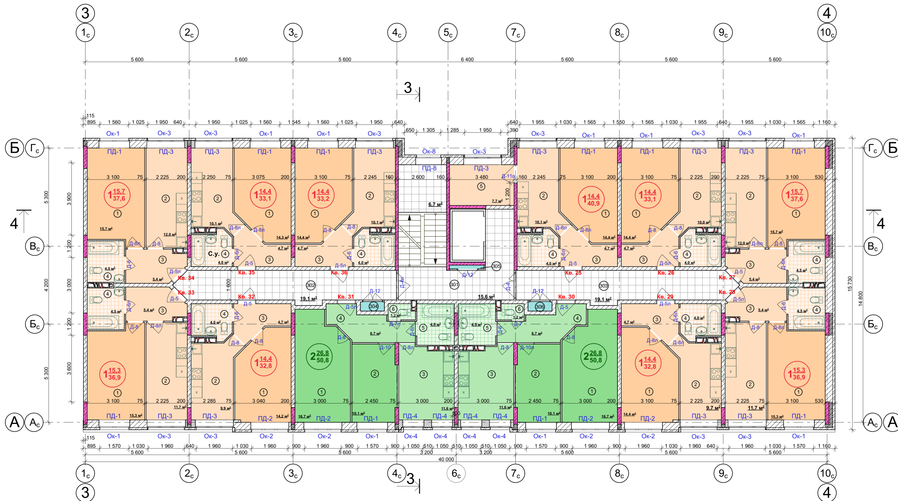
Экспликация помещений 3 этажа (начало)
