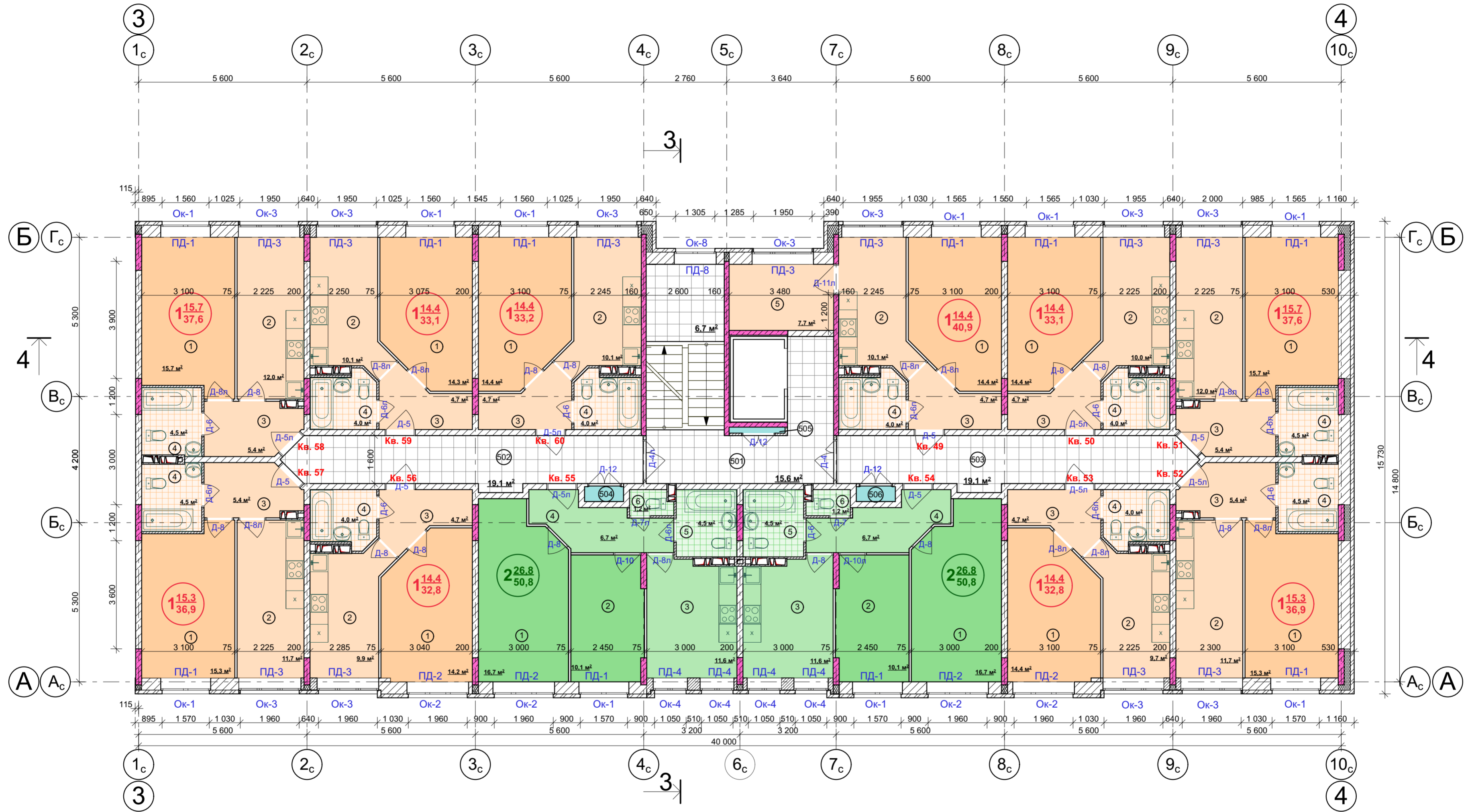
Экспликация помещений 5 этажа (начало)
